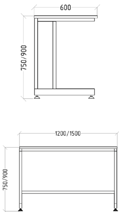
СТОЛ ЛАБОРАТОРНЫЙ
